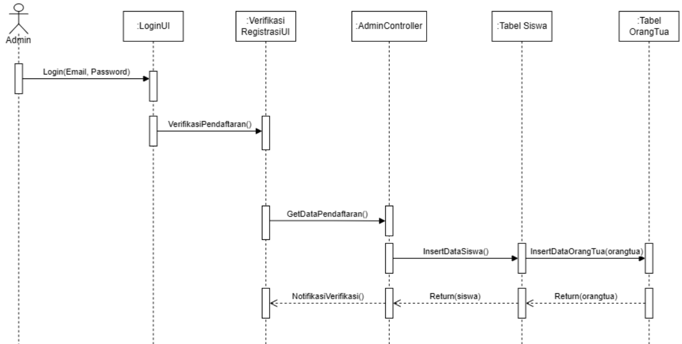
Gambar 3. 39 Sequence Diagram Admin Verifikasi Pendaftaran
