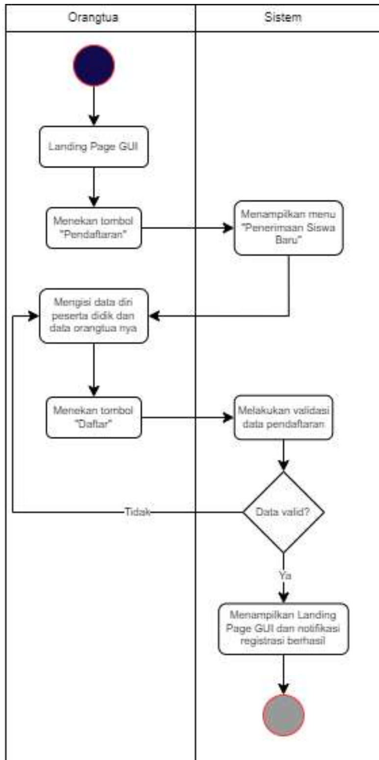
Gambar 3. 4 Activity Diagram Pendaftaran Peserta Didik Baru
