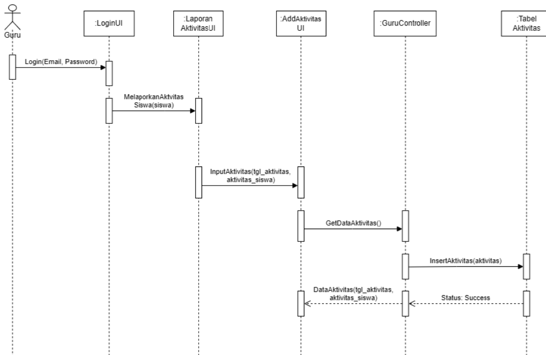
Gambar 3. 34 Sequence Diagram Guru Pelaporan Aktivitas
