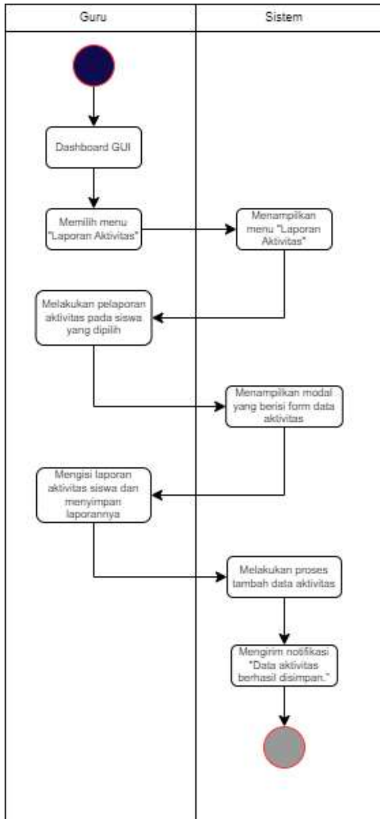
Gambar 3. 6 Activity Diagram Input Laporan Aktivitas Siswa
