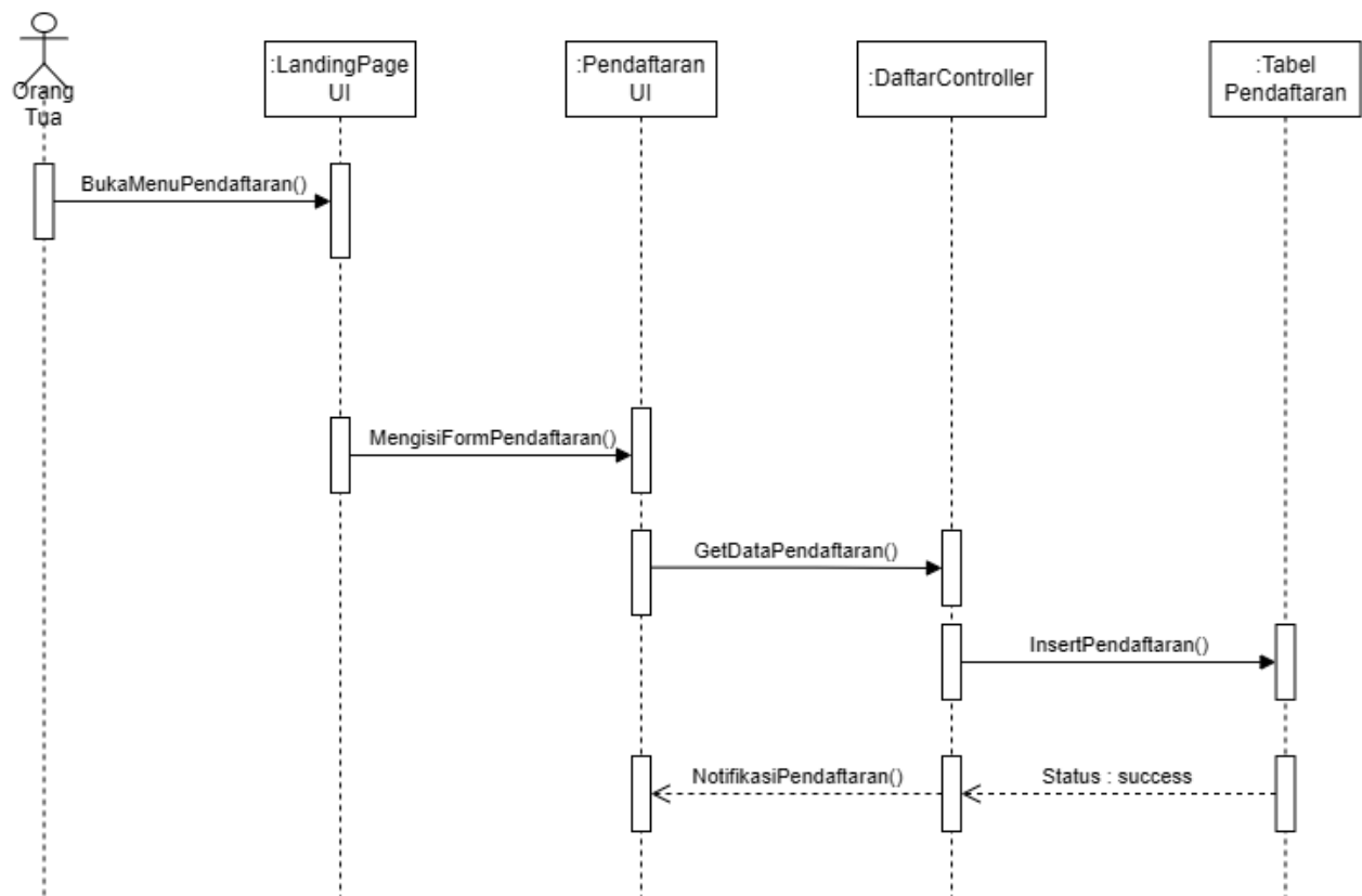
Gambar 3. 38 Sequence Diagram Orang Tua Pendaftaran Siswa
