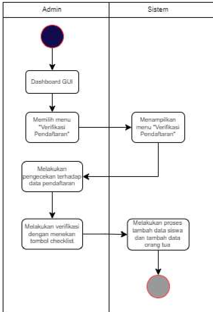
Gambar 3. 5 Activity Diagram Verifikasi Pendaftaran
